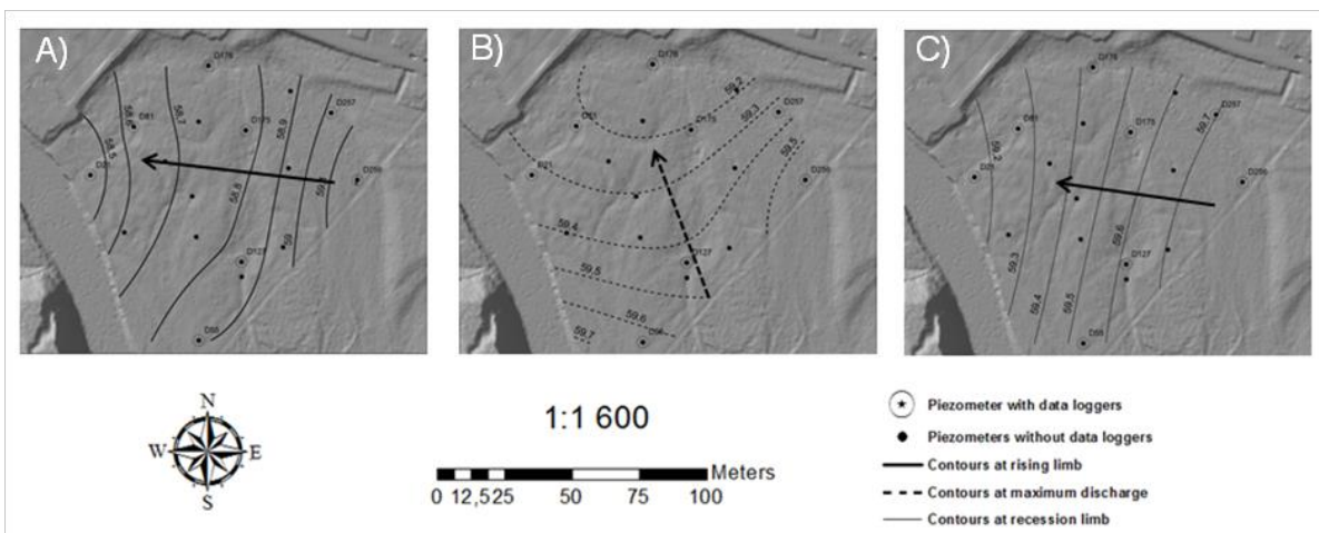
Figure 5.45 Directions de l'écoulement souterrain suggérées par les lignes équipotentiellles durant la plus forte crue survenue du 5 au 12 septembre 2011. A) Directions à 22 \text{ m}^3 \text{ s}^{-1} le 5 e septembre à minuit; B) directions au maximum de crue de 213 \text{ m}^3 \text{ s}^{-1} le 6 septembre à 14h00; C) directions durant la récession à 112 \text{ m}^3 \text{ s}^{-1} le 7 septembre à 13h00 (Cloutier et al. , en prép.).
