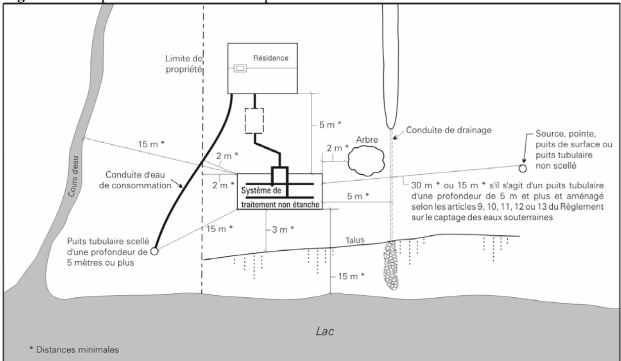
Figure 6.7 Emplacement d'un élément épurateur
