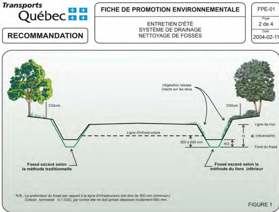
Figure 6.1 Méthode du tiers inférieur pour l'entretien des fossés
