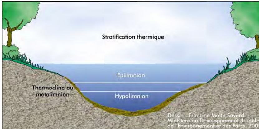
Figure 4.1 Stratification thermique d'un lac en été
