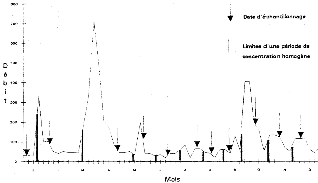
Figure 3 - Périodes de concentration homogène représentées sur l'hydrogramme de la rivière Yamaska à son embouchure pour l'année 1986 (débit en m^3/s )
