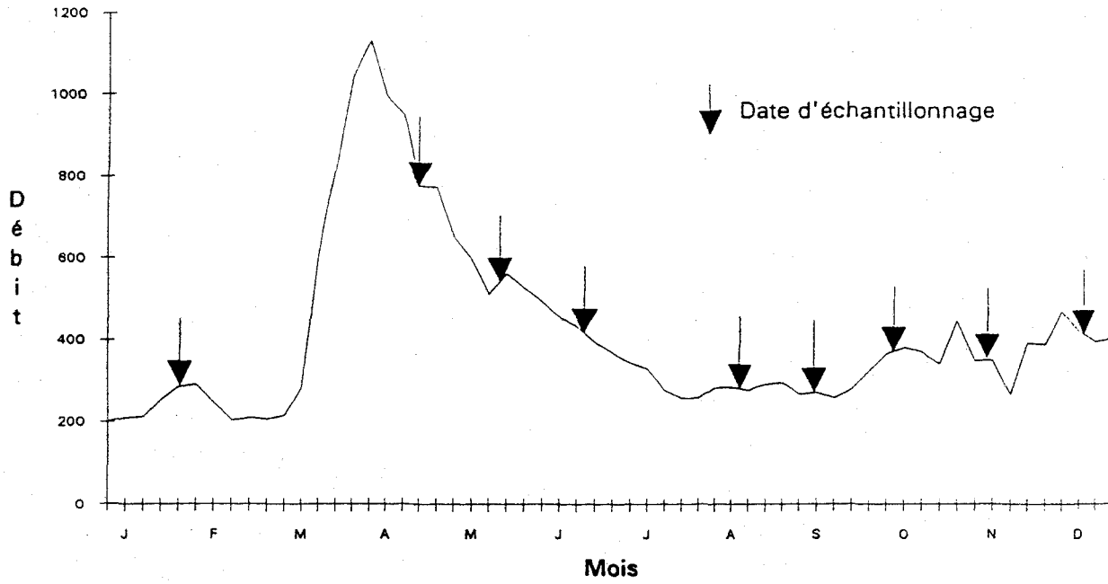
Figure B.3: Hydrogramme de la rivière Richelieu pour l'année 1986 (m 3 /s)
