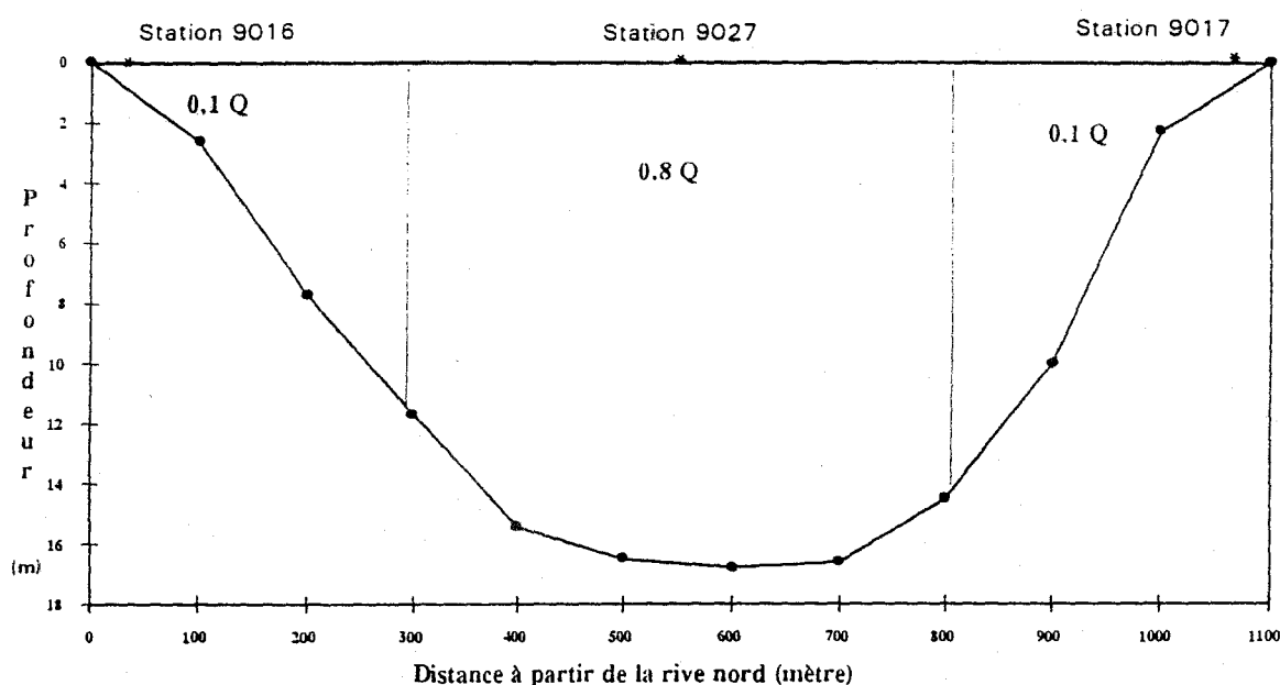
Figure 8 - Profil bathymétrique du fleuve Saint-Laurent et localisation des stations de mesures de qualité de l'eau au transect de Lanoraie
