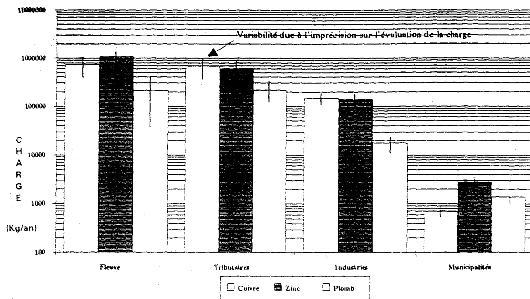
Figure 9 - Bilan de charge pour les trois métaux de référence des quatre principales sources de contamination du lac Saint-Pierre
