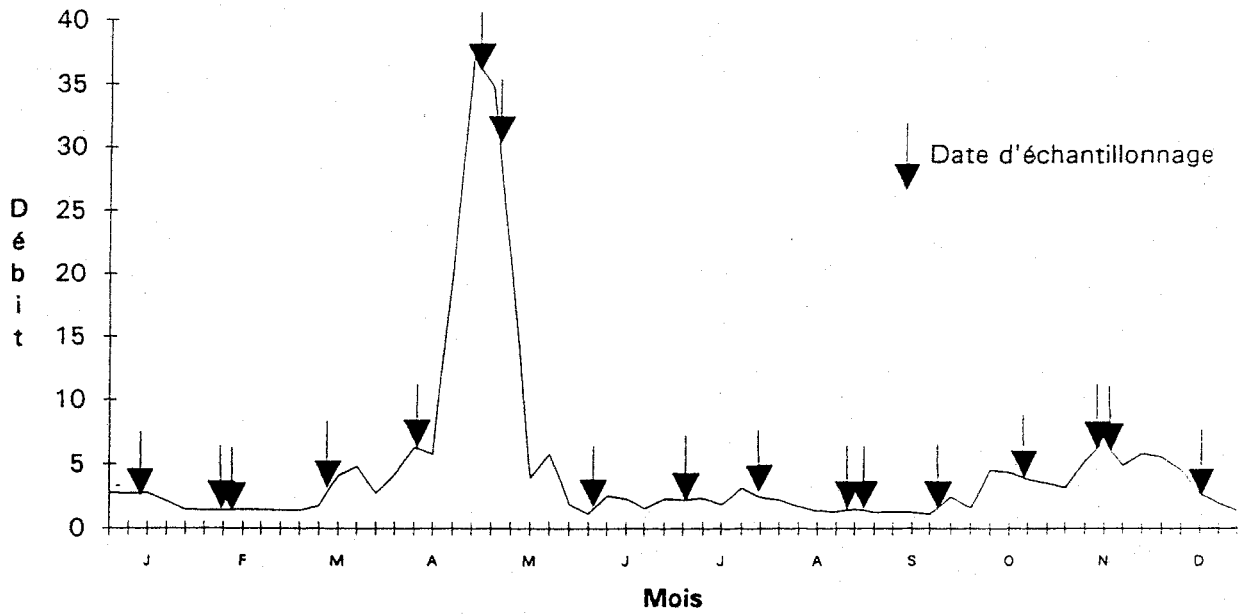
Figure B.4: Hydrogramme de la rivière Bayonne pour l'année 1985 (m 3 /s) (station de débit sur la rivière Maskinongé)
