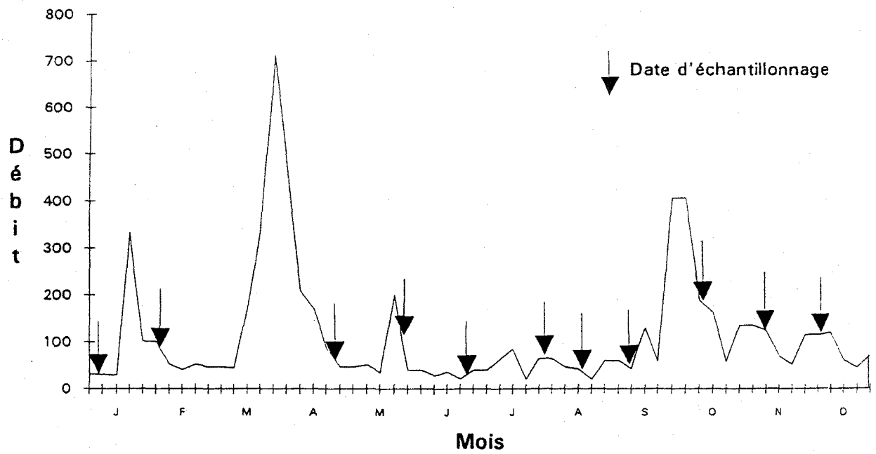
Figure B.2: Hydrogramme de la rivière Yamaska pour l'année 1986 (m 3 /s)
