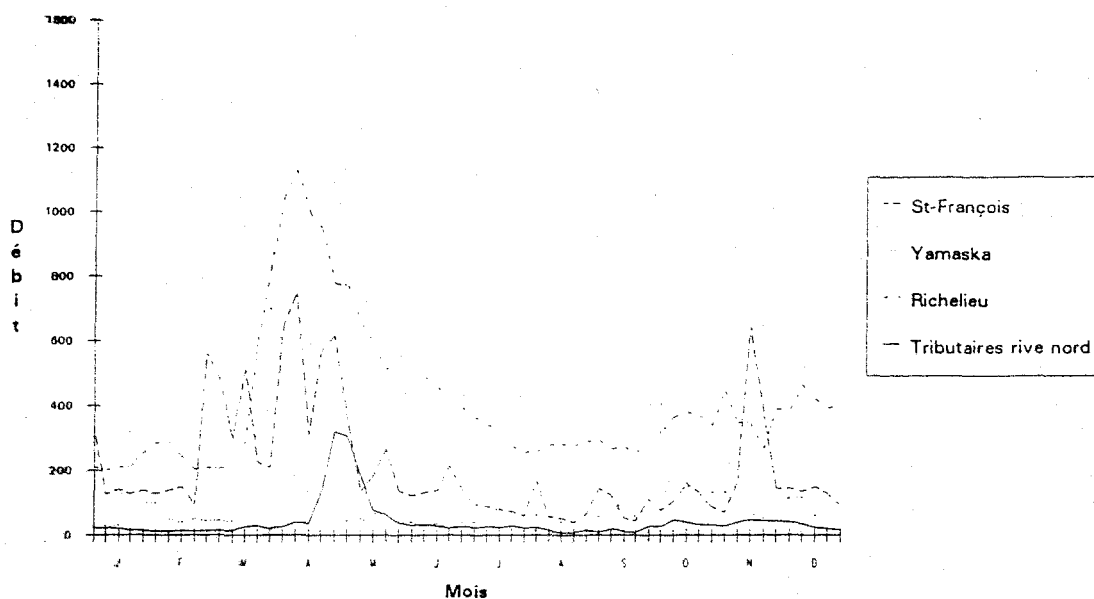
Figure 6 - Hydrogrammes des débits à l'embouchure utilisés pour le calcul des charges en cuivre ( \text{m}^3/\text{s} )
