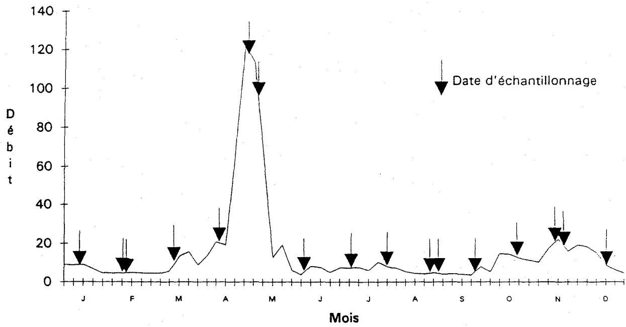
Figure B.5: Hydrogramme de la rivière Maskinongé pour l'année 1985 (m 3 /s)
