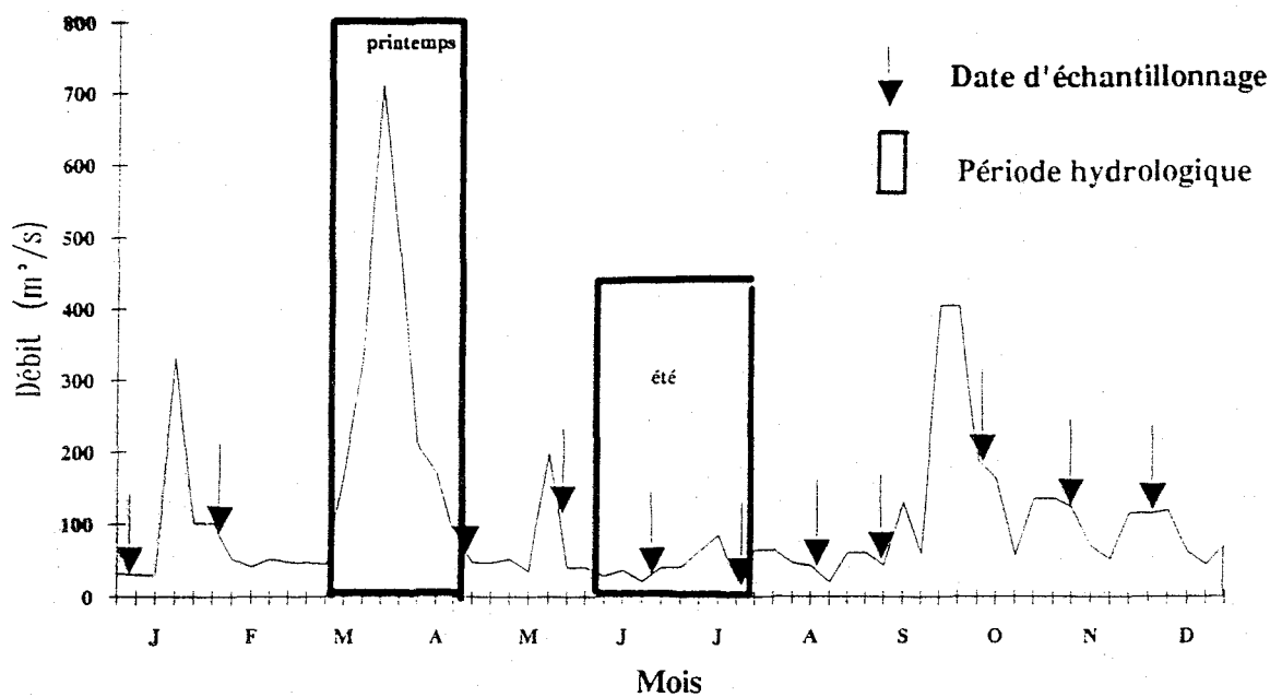
Figure 4 - Saisons printanière et estivale représentées sur l'hydrogramme de la rivière Yamaska à l'embouchure pour l'année 1986 (débit en m^3/s )
