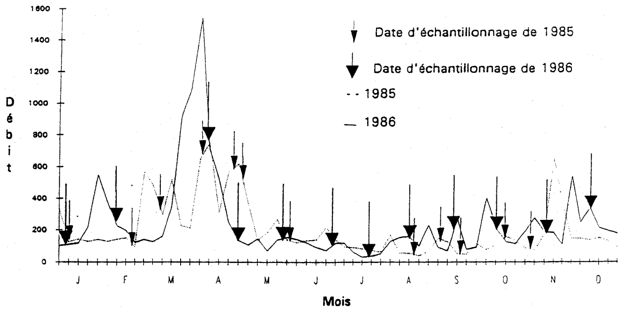
Figure B.1: Hydrogramme de la rivière Saint-François pour les années 1985 et 1986 (m 3 /s)
