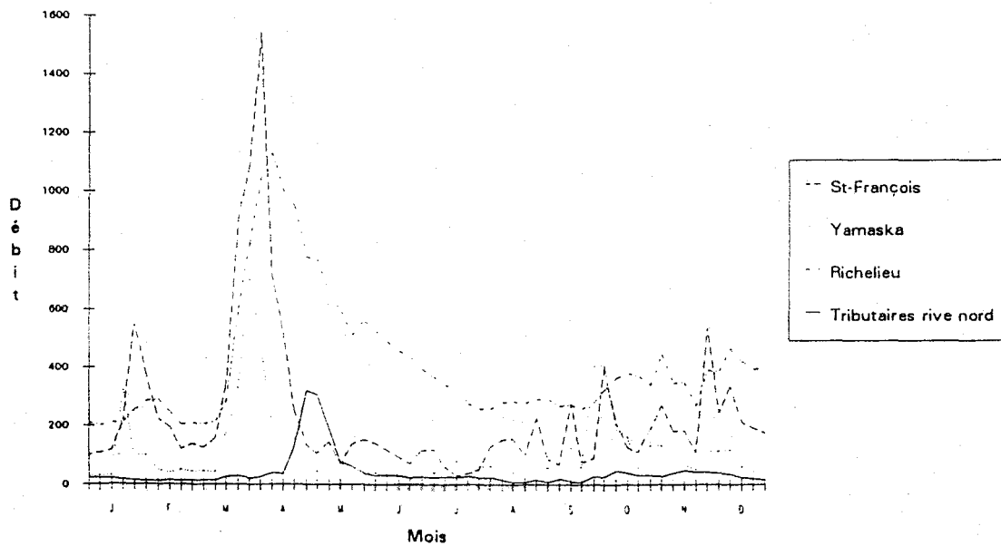
Figure 5 - Hydrogrammes des débits à l'embouchure utilisés pour le calcul des charges en zinc, plomb, nickel, fer, manganèse, cadmium, chrome, et arsenic (m 3 /s)
