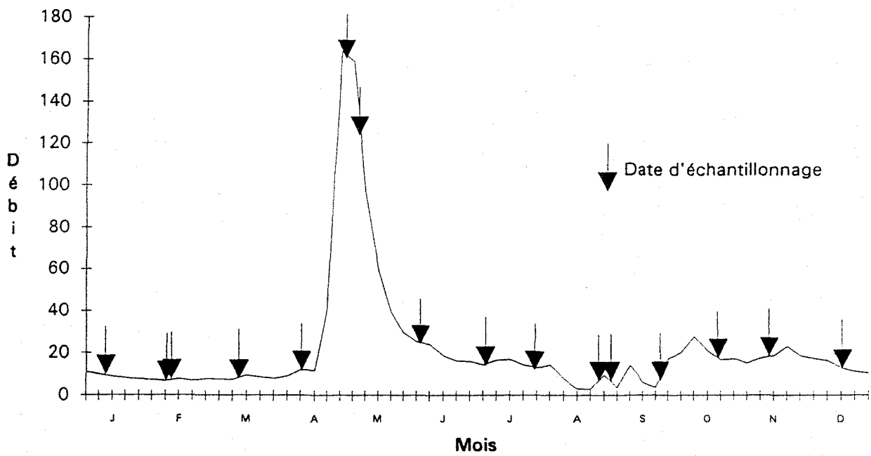
Figure B.6: Hydrogramme de la rivière du Loup pour l'année 1985 (m 3 /s)
